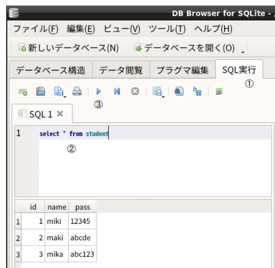
図 6.5 SELECT の実行
