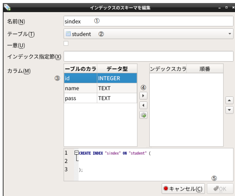
図 6.9 インデックスの設定画面
