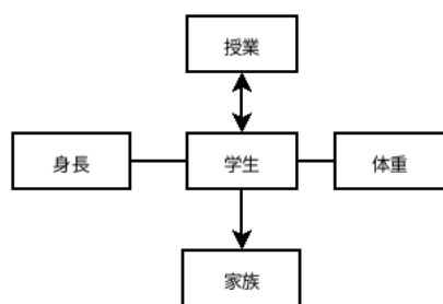
図 6.6 ER 図の例
